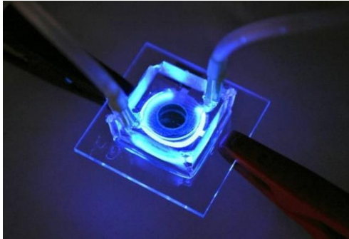
Abbildung 1: Prototyp eines OLED-OPD-Chips zur Fluoreszenzdetektion.
